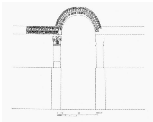
Slika 48 Idejna rekonstrukcija trabeacije oltarne ograde sv. Marije na Poljudu (Matetić, 2002: 282)
