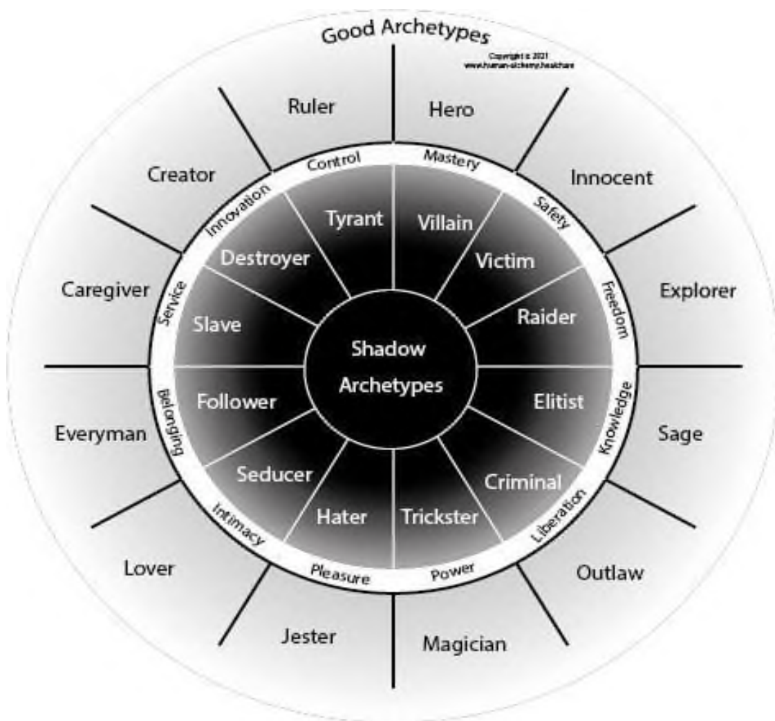
Slika 1 Dvovidnost arhetipa. 10
