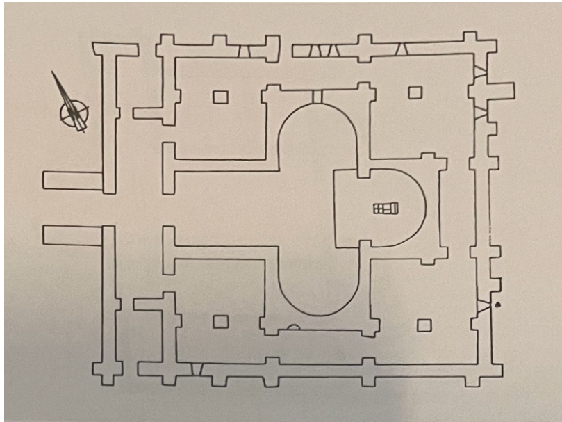
Slika 30. Tlocrt crkve
