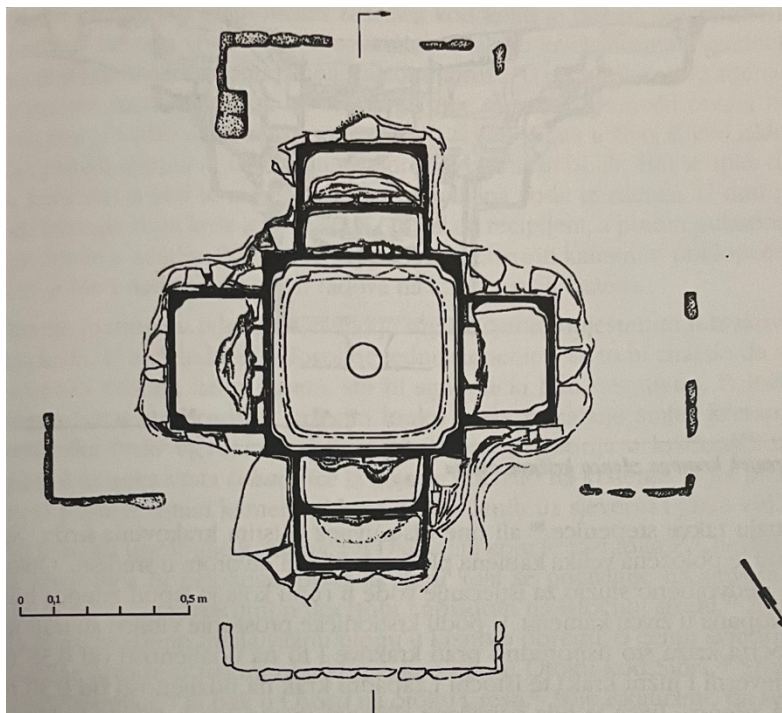
Slika 26. Tlocrt krsnog zdenca križnog oblika
