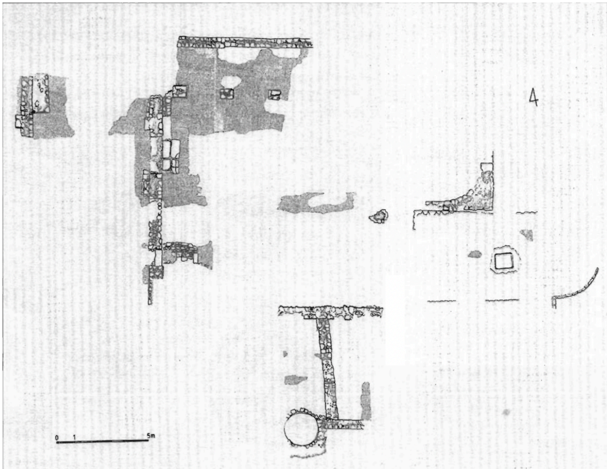
Slika 27. Tlocrt ranokršćanskih ostataka
