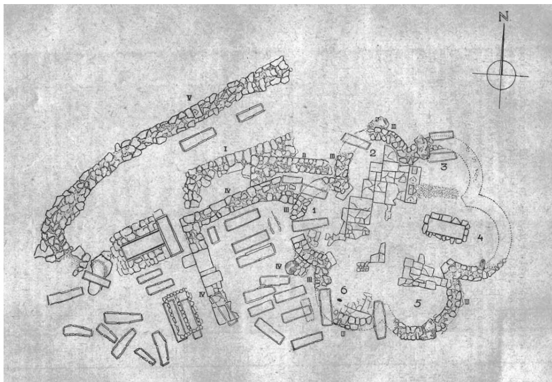
Slika 12. Tlocrt crkve s ostacima drugih objekata
