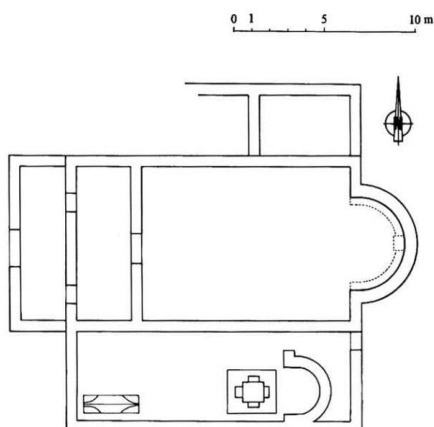
Slika 14. Tlocrt crkve (preuzeto: OŽANIĆ ROGULJIĆ, 2008)
