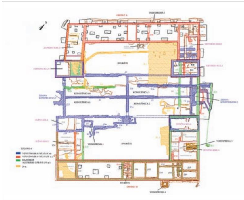
Slika 68. Tlocrt Kvartera
