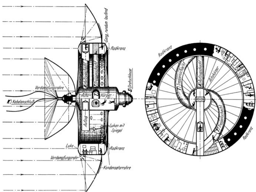
Prilog 8. Načrt stambenog kola. Lijevo: aksijalni presjek; Desno: strana koja je stalno okrenuta prema Suncu, bez zbirnoga zrcala, djelomično u presjeku. 266
