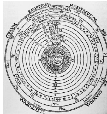
Slika 2 - Geocentrični sustav iz Ptolemejeva Almagesta
