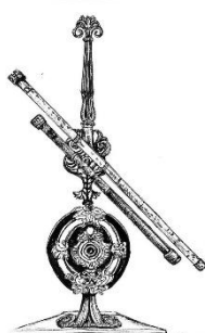
Slika 5 - Galilejev teleskop
