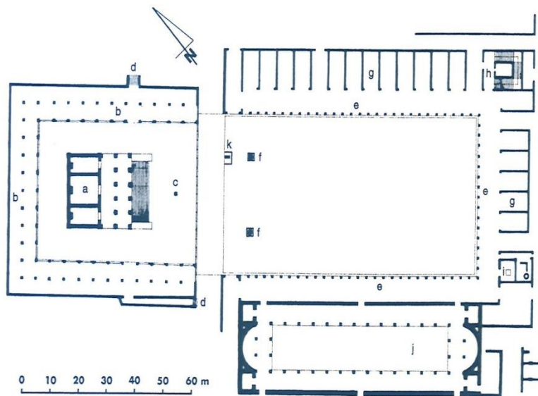
Sl. 94. Kompleks foruma i kapitolija, Zadar ( Iader ) nakon završetka izgradnje: a) kapitolijski hram s trodielnom celom; b) dvostruki trijem oko kapitolija; c) žrtvenik ispred hrama; d) bočni prilazi na kapitolij; e) jednostruki trijem s lodom oko foruma; f) monumentalni ukrasni stupovi; g) niz taberni s dvije strane foruma; h) ugao-ni sklop taberni, stubište za uspon na lodu trijema; i) nimfej s javnom česmom i latrinom; j) severijanska bazilika; k) zdenac; Suić; položaj zdenca prema Fadić 1986a
