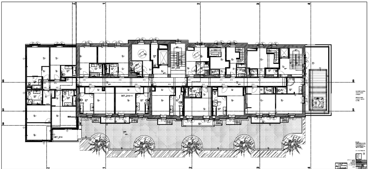
Slika 21. Tlocrt prvog kata (novo stanje) Hotela Park, Emil Šverko/Atelier Šverko i Šverko
