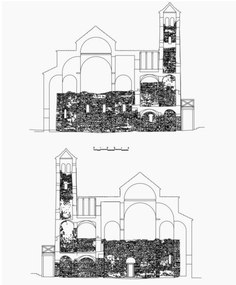
Slika 54. Uzdužni presjek s prikazanim ostacima i pretpostavljenim izvornim izgledom (Milošević/Peković) (Preuzeto: Marasović, Tomislav, 2006.)
