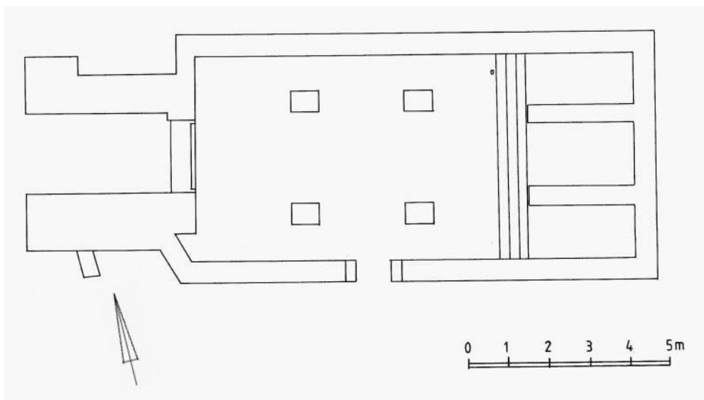
Slika 44. Pretpostavljeni izvorni tlocrt crkve (prema M. Zekanu) (Preuzeto: Marasović, Tomislav., 2006.)
