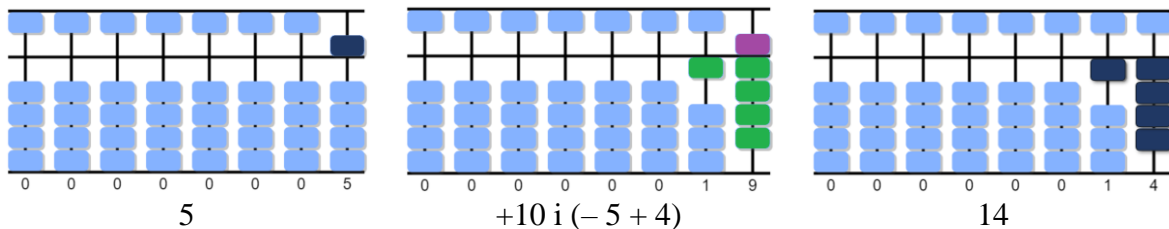
Slika 57. Zbrajanje 5 + 9
