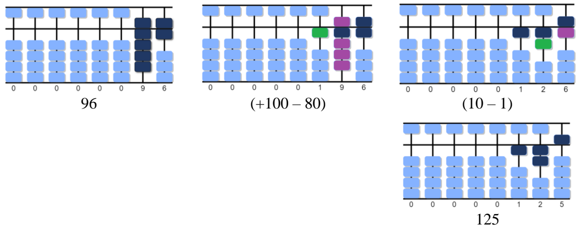
Slika 41. Zbrajanje 96 + 29
