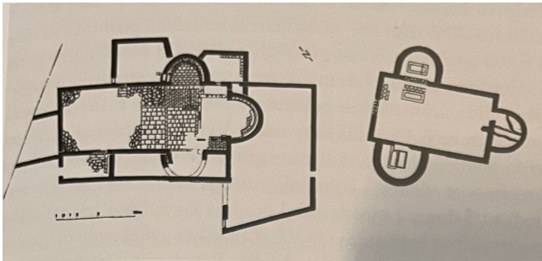
Slika 37. Plan crkvenog kompleksa (crkva i memoria)
