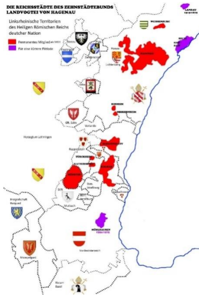
Slika 8. Décapole Elzasa
